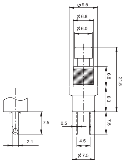
Part N° shown: 5RS3-ST1
